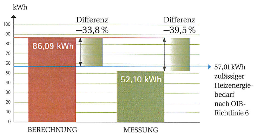
Durchschnittlicher Heizenergiebedarf bestehender Blockhäuser
